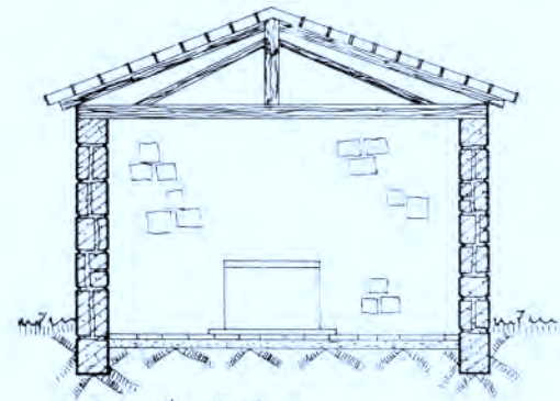
Sección A-B
