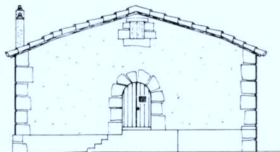
ALZADO FRENTE
