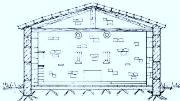
Sección A-B
