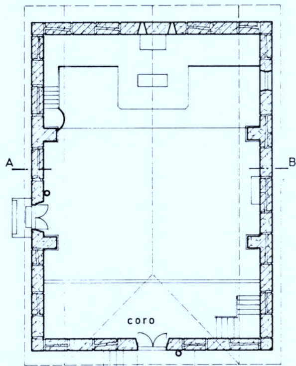
PLANTA
